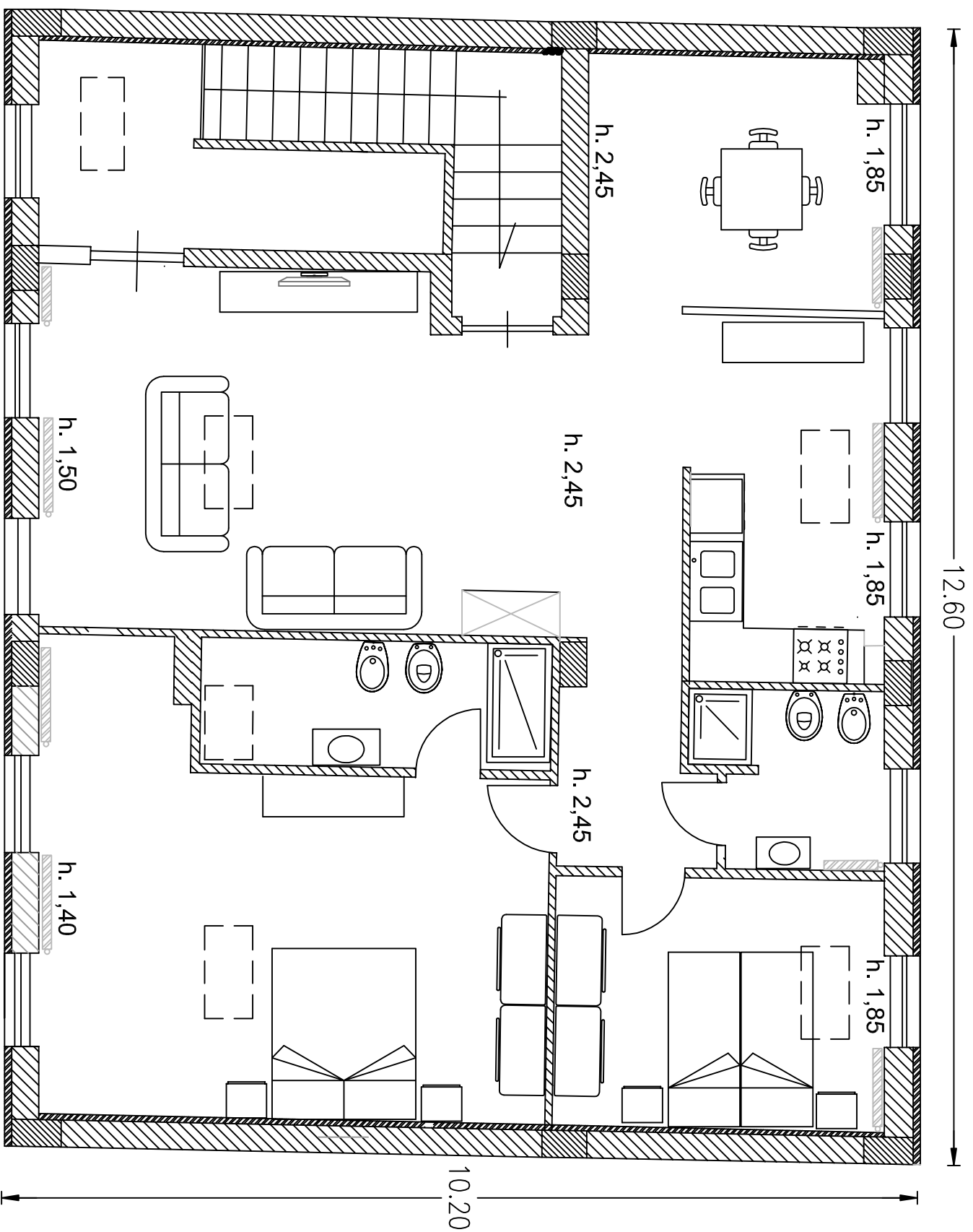
Pianta Piano II° "La Betulla"
